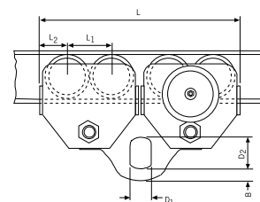
Modèle HTG 20000 kg
