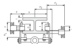
Modèle HTP/G 500 - 5000 kg, avec frein de parking
