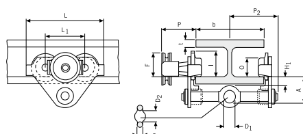
Modèle HTP/G 500 - 5000 kg
